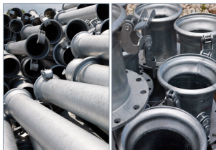
Быстроразъемные трубные фитинги и муфты
